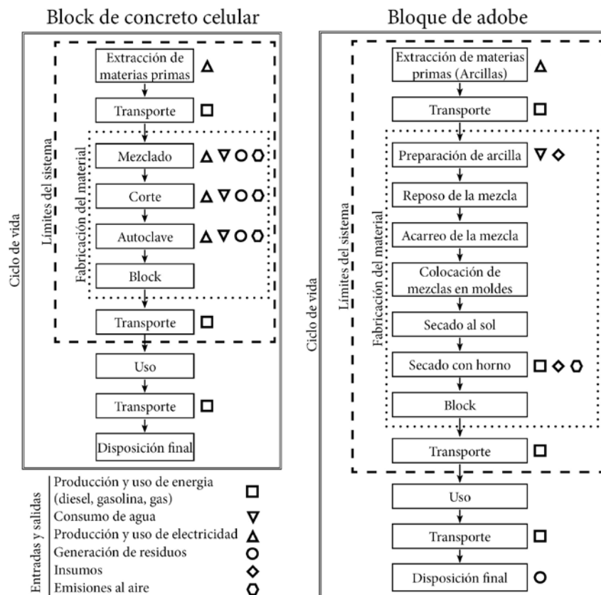
Imagen 1: Diferencias en el ACV entre un bloque de concreto celular y el adobe con las respectivas entradas de recursos y salida de desechos y emisiones (elaborado a partir de Güereca Hernández et al., 2016)
